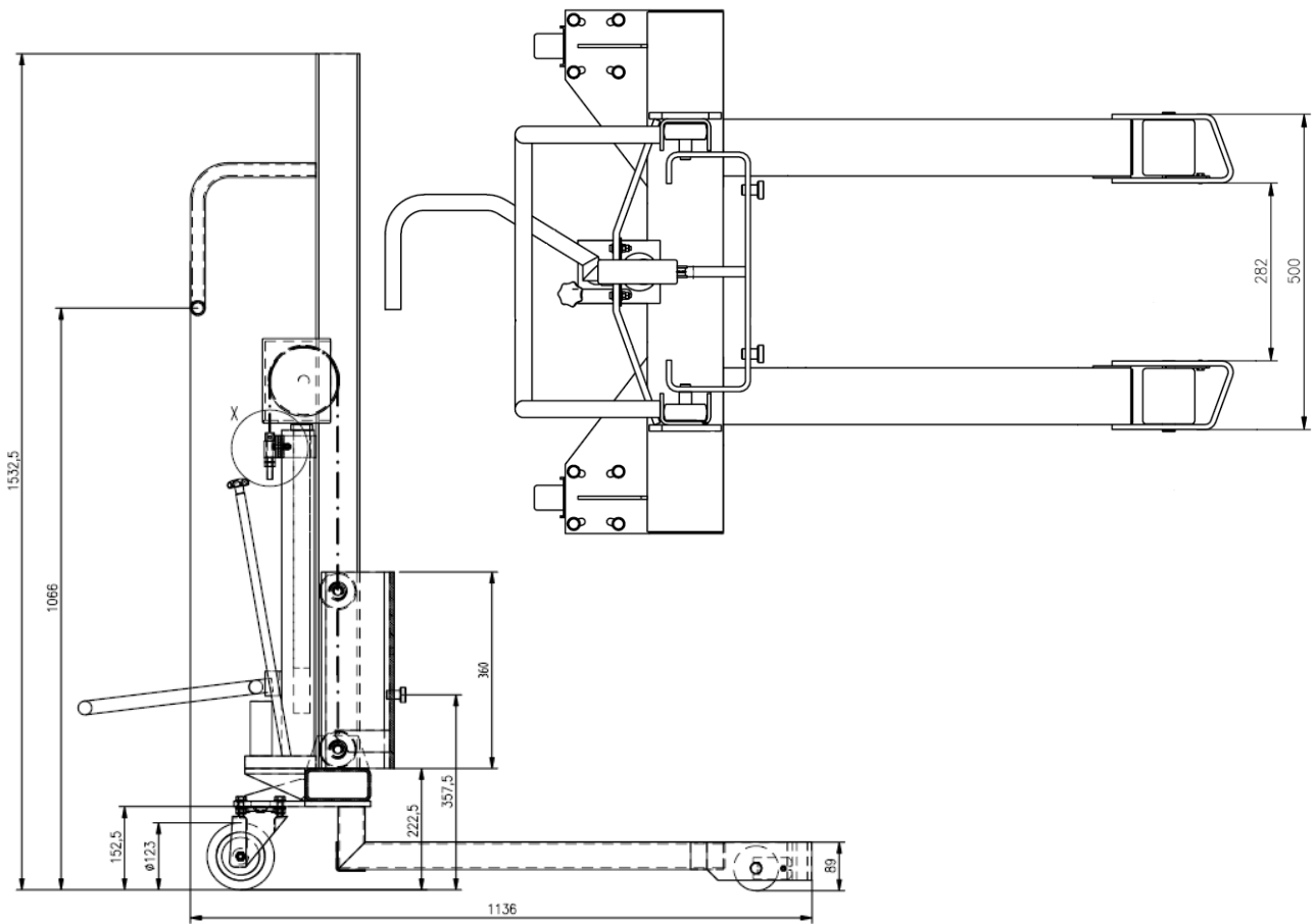
DENIOS Fasslifter Servo Typ FL 8-xxx; FW 8 (Fahrwerke für alle Versionen: FL-M, FL-K, FW)
